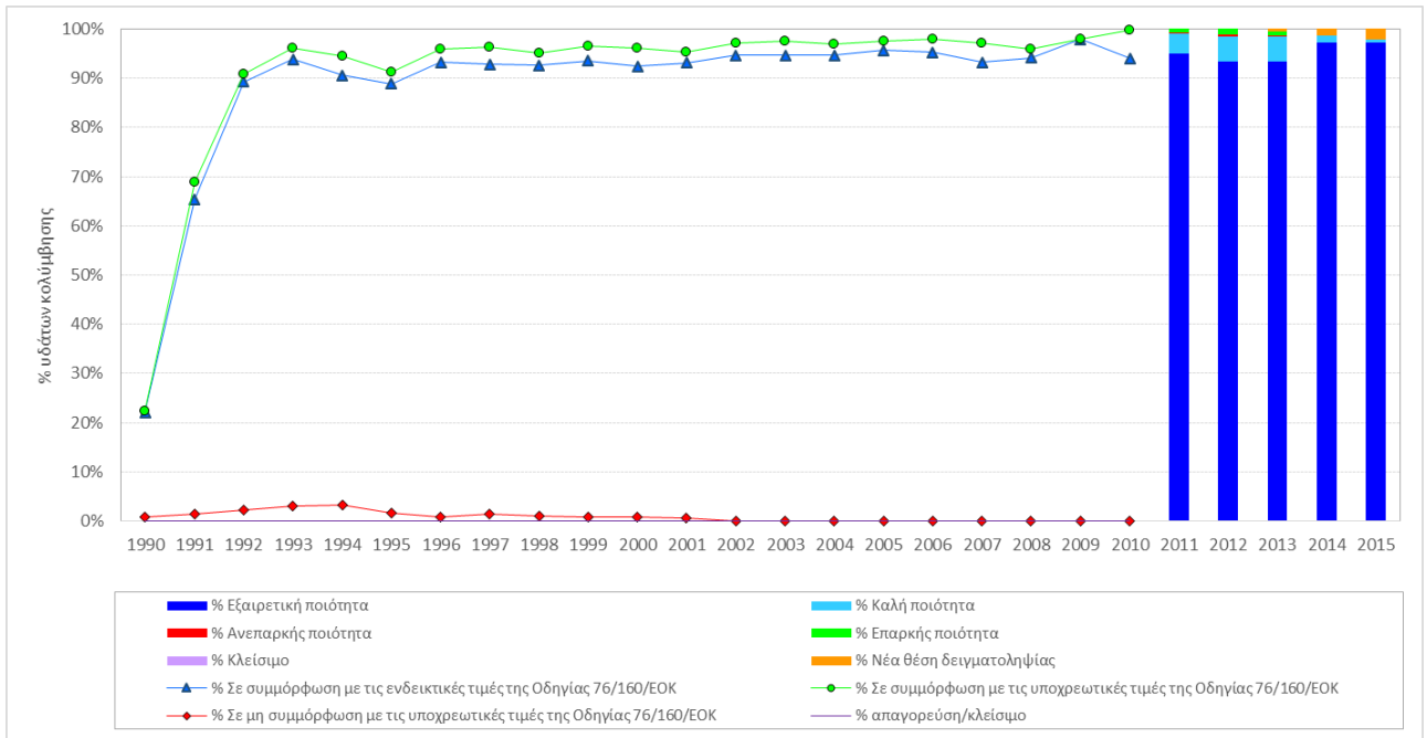
Γράφημα 4 : Ταξινόμηση των παράκτιων υδάτων κολύμβησης της Ελλάδας από το 1990 έως το 2015
