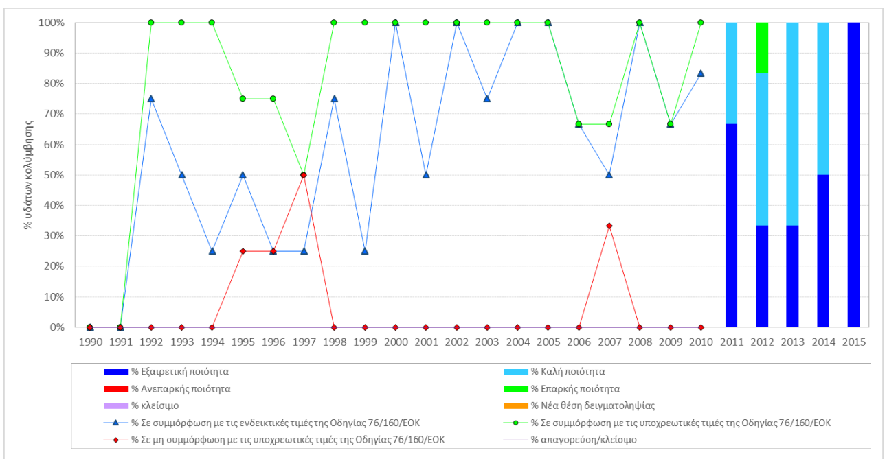
Γράφημα 5: Ταξινόμηση των εσωτερικών υδάτων κολύμβησης της Ελλάδας από το 1990 έως το 2015
