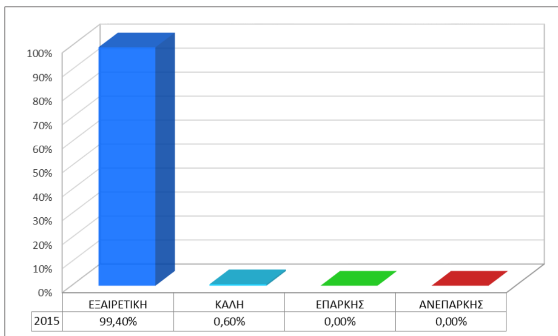
Γράφημα 1 : Ταξινόμηση των υδάτων κολύμβησης σύμφωνα με την Οδηγία 2006/7/ΕΚ με έτος αναφοράς 2015
