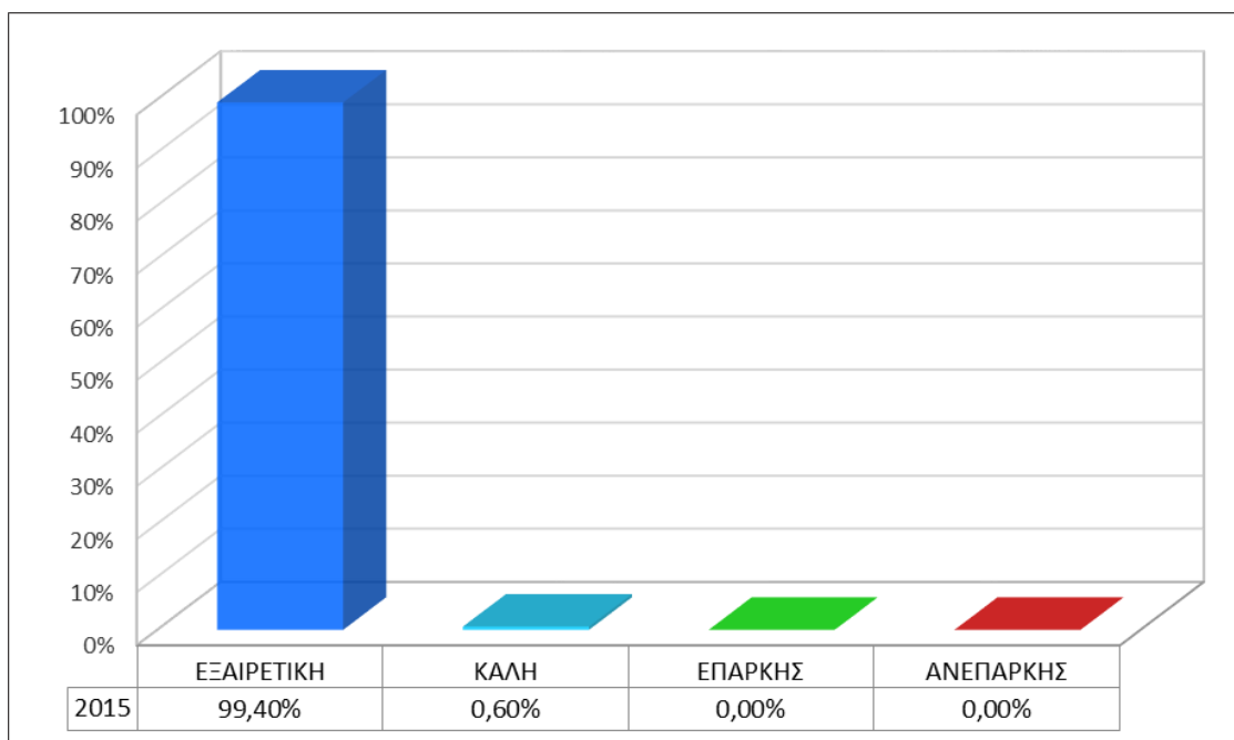
Γράφημα 2 : Ταξινόμηση των παράκτιων υδάτων, σύμφωνα με την Οδηγία 2006/7/ΕΚ, με έτος αναφοράς 2015
