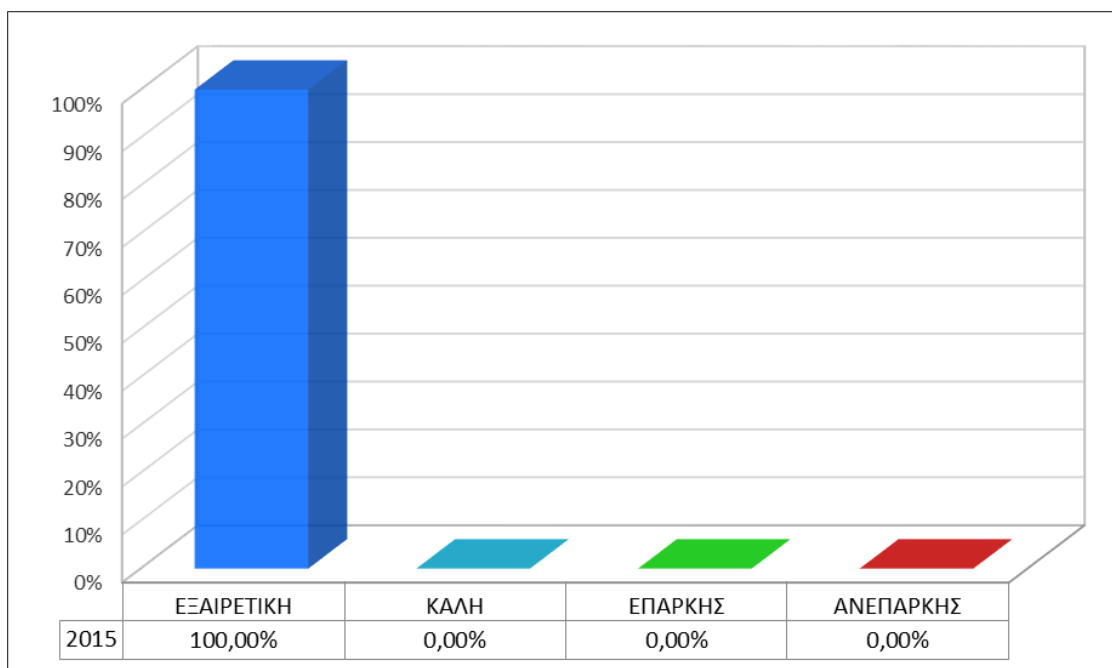
Γράφημα 3 : Ταξινόμηση των εσωτερικών υδάτων κολύμβησης σύμφωνα με την Οδηγία 2006/7/ΕΚ με έτος αναφοράς 2015
